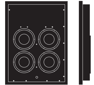
DFS100-75 Subwoofer H:1000 W:750 D:133mm
